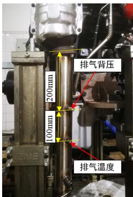
图A.4 排气背压与排气温度测量位置
