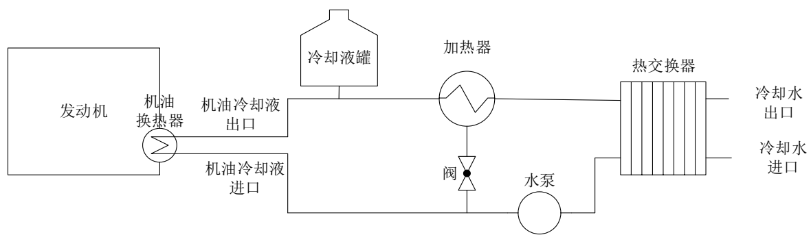
图 B.3 典型的机油温控系统示意图
