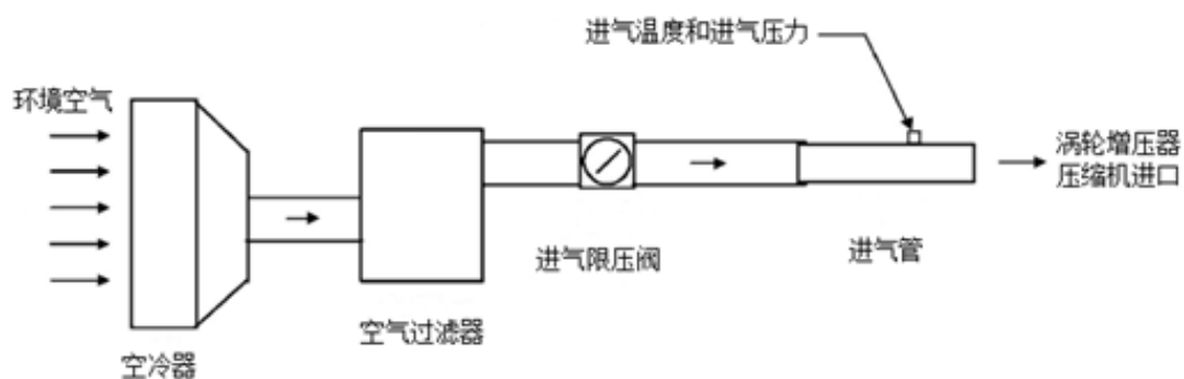
图 B.1 典型的进气系统示意图
