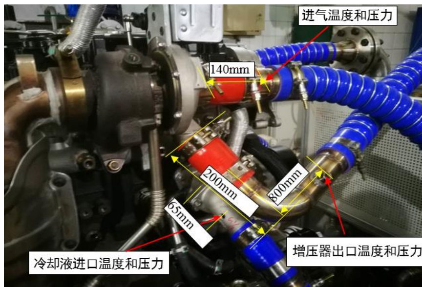
图A.3 冷却液进口、增压器出口温度与压力测量位置
