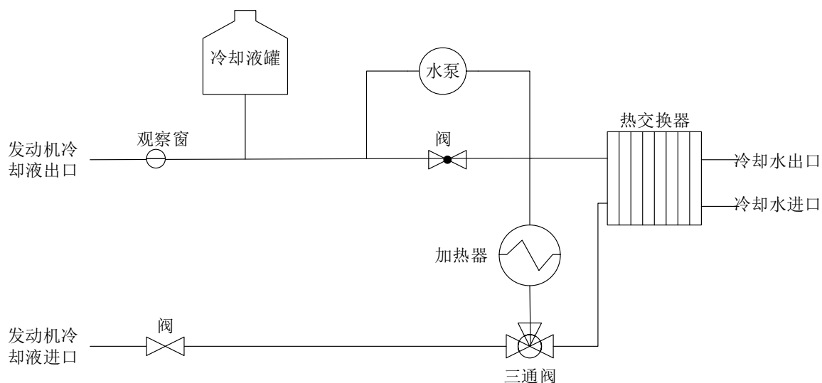
图 B.2 典型的发动机冷却系统示意图
