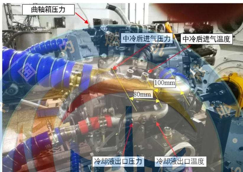
图A.1 冷却液出口、中冷后进气温度与压力测量位置
