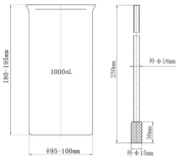
图 2 烧杯及气体扩散管
