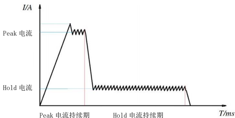
图 1 喷射阀驱动电流示意图
